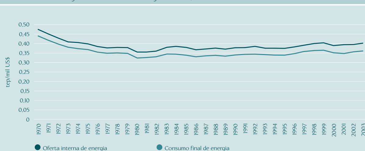
GRÁFICO 4 • Medidas de intensidade no uso de energia, calculadas a partir de dados de oferta de energia e consumo de energia – Brasil, 1970 a 2003
